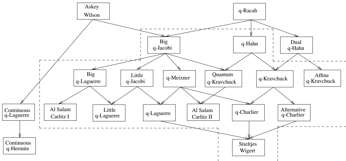
Figura A.1: Ejemplos de las tablas de Askey y de Hahn (separados por --) considerados en esta memoria
