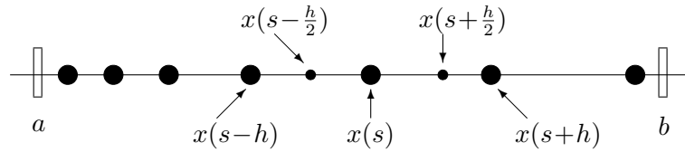
Figura 2.1: Discretización en una red no uniforme x(s)
